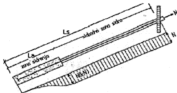
Dijagram promjene zatežuće sile sidra
